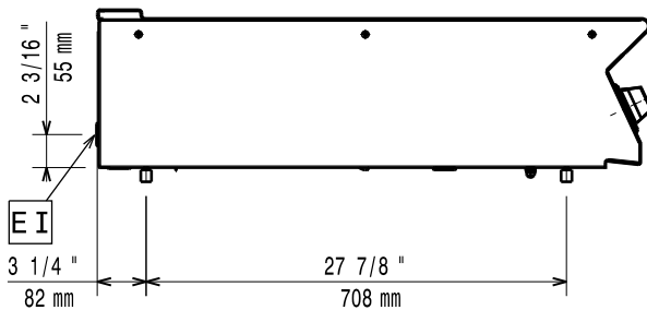
Oldalnézet
